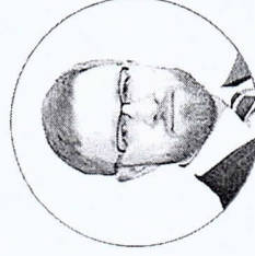
Малькевич
